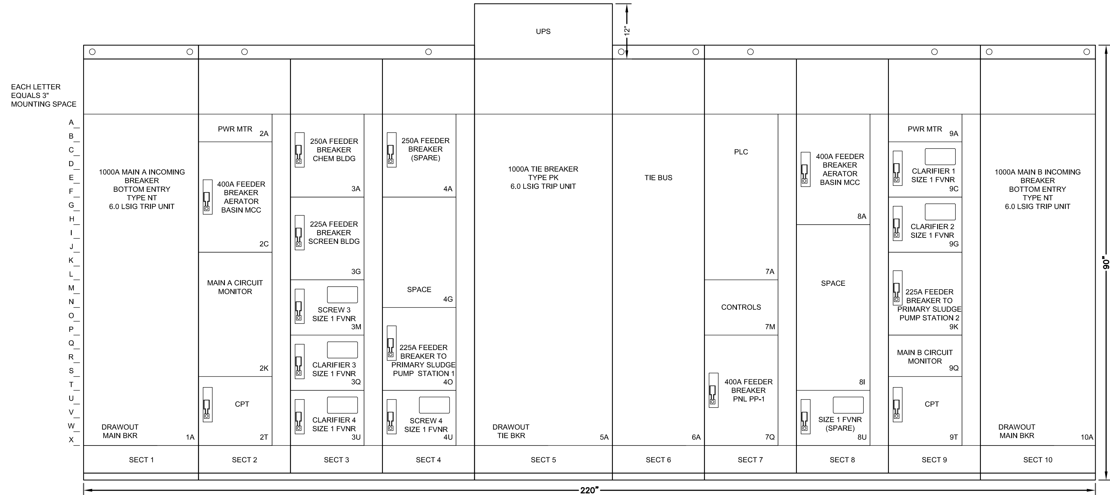
2 MCC-7 - MCC ELEVATION SCALE: NONE
